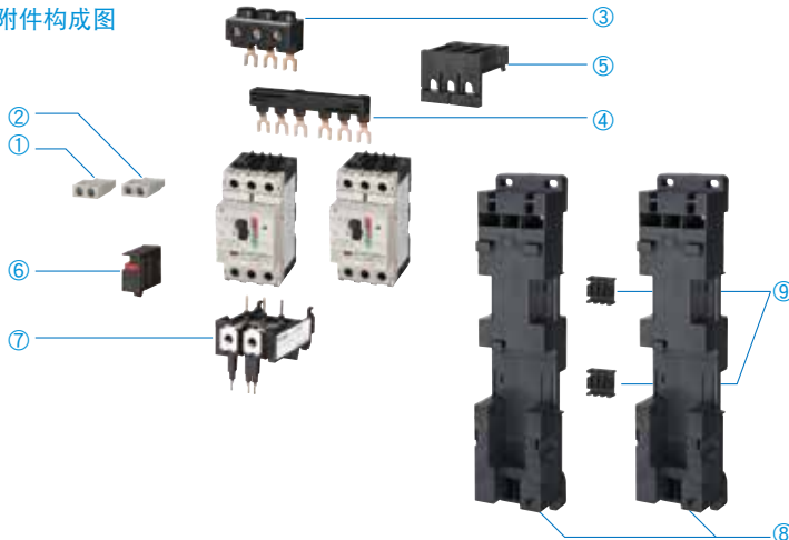
●附件构成图
